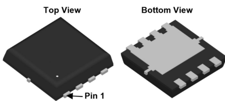
PDFN3x3-8L
